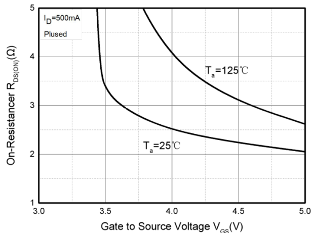
RDS(ON)— V_{GS}
