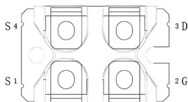
SOT-227
